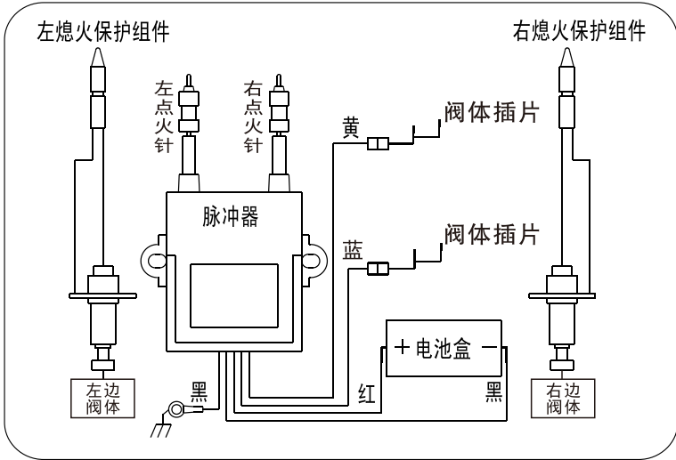
燃气灶内部连线示意图（热电偶保护）
